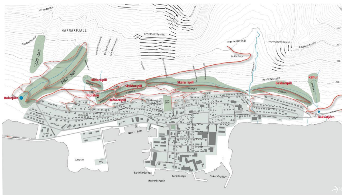
Mynd 18. Snjóflóðavarnargarðar ofan Siglufjarðar.
